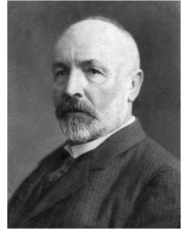
Georg Cantor
